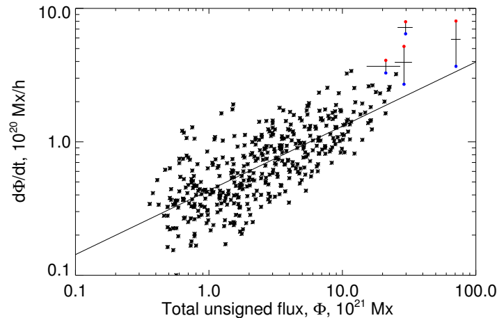
Рис. 3. Зависимость скорости всплытия магнитного потока ( d\Phi/dt , 10^{20} Мкс/ч) от суммарного беззнакового магнитного потока ( \Phi , 10^{21} Мкс) активной области. Черными звездами отмечены магнитные структуры, исследованные в работе Kutsenko et al. (2019), крестами – усредненное расположение АО, рассматриваемых в данной работе. Для каждой из четырех добавленных АО горизонтальные сегменты обозначают разницу между максимальными потоками \Phi_1 и \Phi_2 . Красными кружками отмечены значения максимальной мгновенной скорости всплытия магнитного потока, синими – значения его средней скорости
