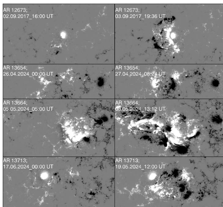
Рис. 1. Изображения рассмотренных активных областей NOAA 12673, 13654, 13664 и 13713. Слева представлены магнитограммы на момент начала всплытия мультиполярной структуры, справа – на момент времени с максимальной мгновенной скоростью всплытия. Черный и белый цвет соответствуют плотности магнитного потока -800 и 800 \text{ Мкс см}^{-2} соответственно. Длина каждой магнитограммы 344'' или около 250 \text{ Мм} . Северный полюс находится сверху, запад – справа
