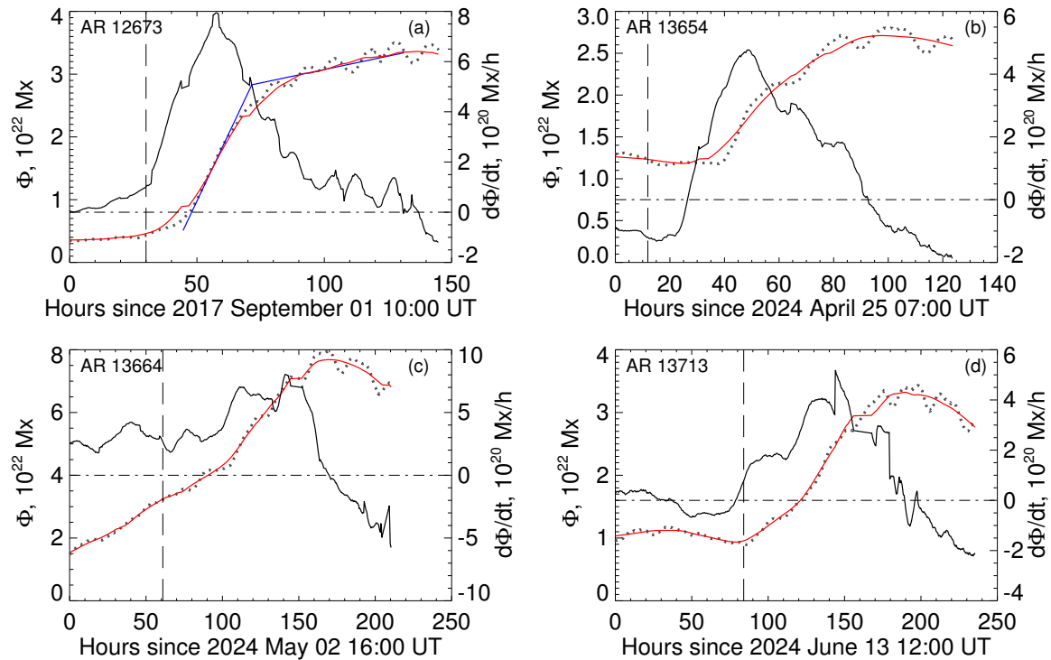
Рис. 2. Изменение суммарного магнитного потока ( \Phi , 10^{22} Мкс, левая ось) и мгновенной скорости всплывания потока ( d\Phi/dt , 10^{20} Мкс/ч, правая ось) со временем. Серая пунктирная линия показывает изначальные значения потока, красная сплошная кривая – сглаженные. Черная сплошная линия обозначает изменение мгновенной скорости всплывания потока. Синяя кривая на панели (a) показывает пример полученной кусочно-линейной функции для вычисления средней скорости всплывания магнитного потока. Горизонтальная штрихпунктирная прямая показывает нулевой уровень для мгновенной скорости всплывания потока. Вертикальной штриховой линией обозначено примерное время начала активного всплывания основной мультиполярной структуры АО. Время указано в часах
