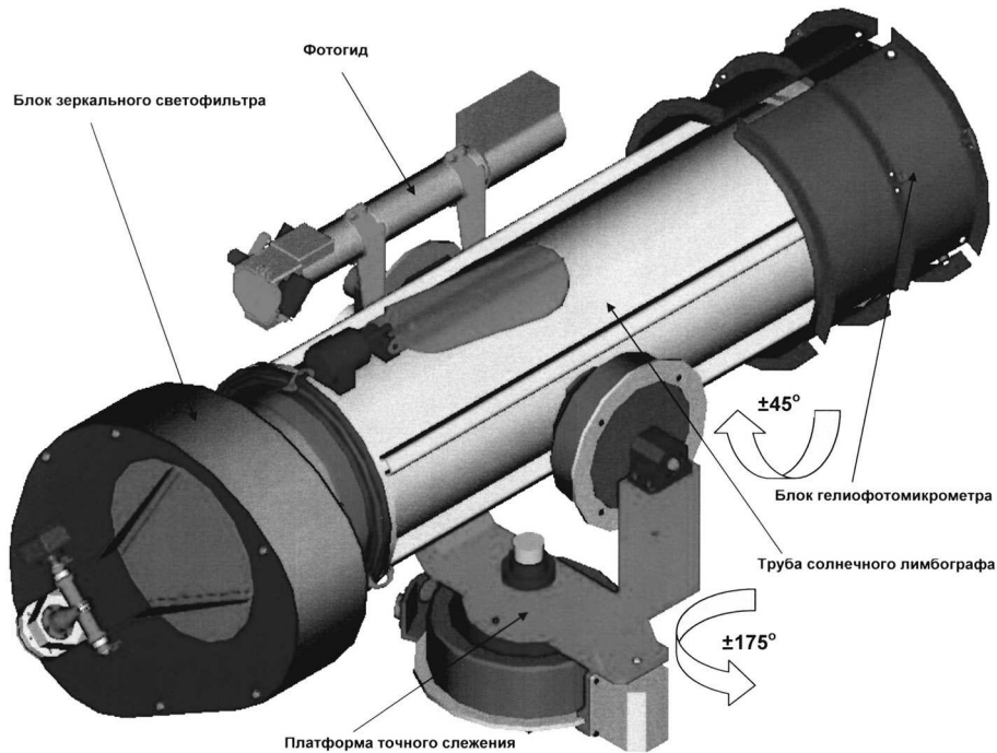
Рис. 3. Общий вид блока оптики и механики (БОМ) комплекса СЛ-200
