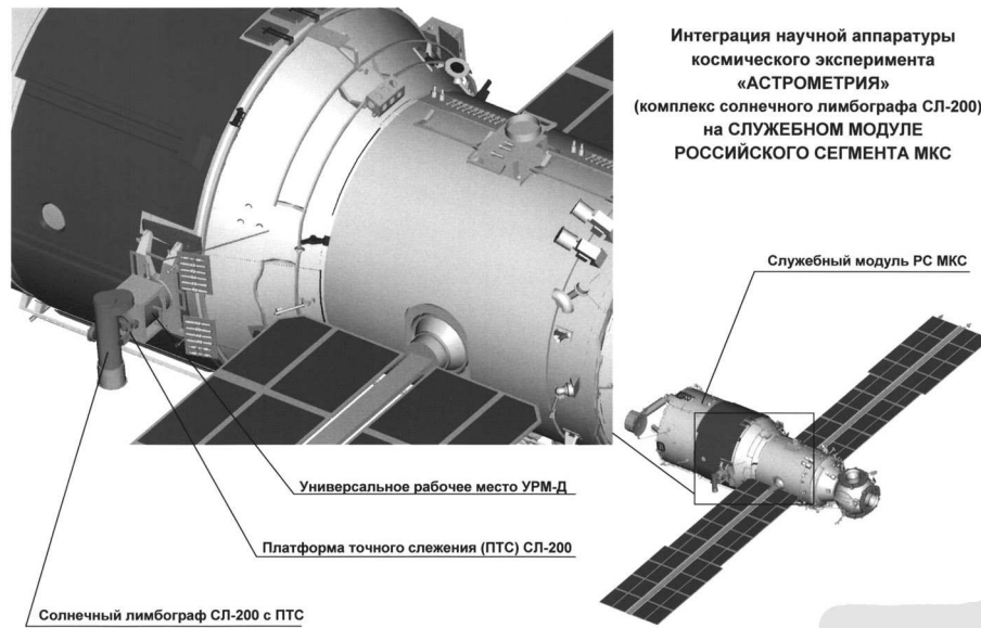
Рис. 5. Размещение комплекса научной аппаратуры СЛ-200 проекта «Астрометрия» на СМ РС МКС
