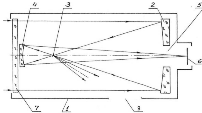
Рис. 1. Оптическая схема солнечного лимбографа с ходом лучей для осевого пучка системы, где 1 – инваровый корпус (труба) лимбографа, 2 – вогнутое эллипсоидальное главное зеркало \varnothing_{\text{св}} 200 мм из карбида кремния ( \lambda/50 ) с центральным отверстием 5 \varnothing 49 мм, 3 – плоское непрозрачное теплозащитное зеркало – “луна” – эллиптической формы с угловым диаметром не менее 1800'' с центральными двумя отверстиями, 4 – вторичное вогнутое эллипсоидальное зеркало \varnothing_{\text{св}} 44 мм из карбида кремния ( \lambda/50 ), 6 – регистрирующее фотоприемное устройство (специальная ПЗС-матрица) \varnothing 50 мм в фокальной плоскости лимбографа, 7 – зеркальный свето(спектро)делительный фильтр (ЗСВФ) из кварцевого стекла КУ-1 \varnothing_{\text{св}} 188 мм ( \lambda/50 ), определяющий апертуру системы при наблюдениях Солнца, являясь ее входным зрачком, 8 – отверстие в корпусе лимбографа. При наблюдении звезд ЗСВФ выводится из светового пучка и входным зрачком оптической системы служит диафрагма диаметром 200 мм.
