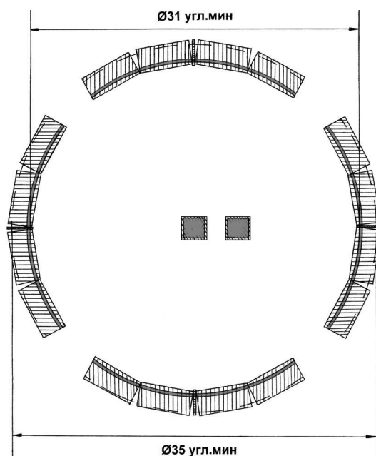
Рис. 4. Расположение матриц ПЗС на панели фотоприемного устройства
